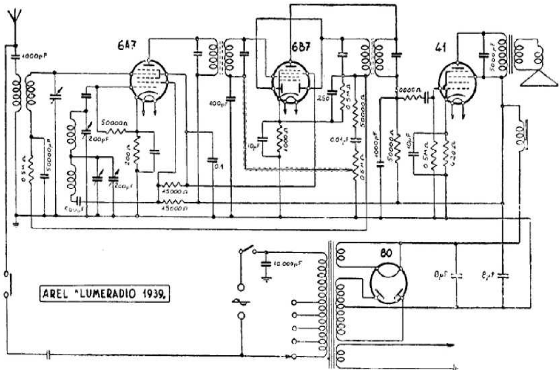
AREL. — Mod. « Lumeradio ». — Produzione 1938-39. — Media frequenza: 450 kHz.
